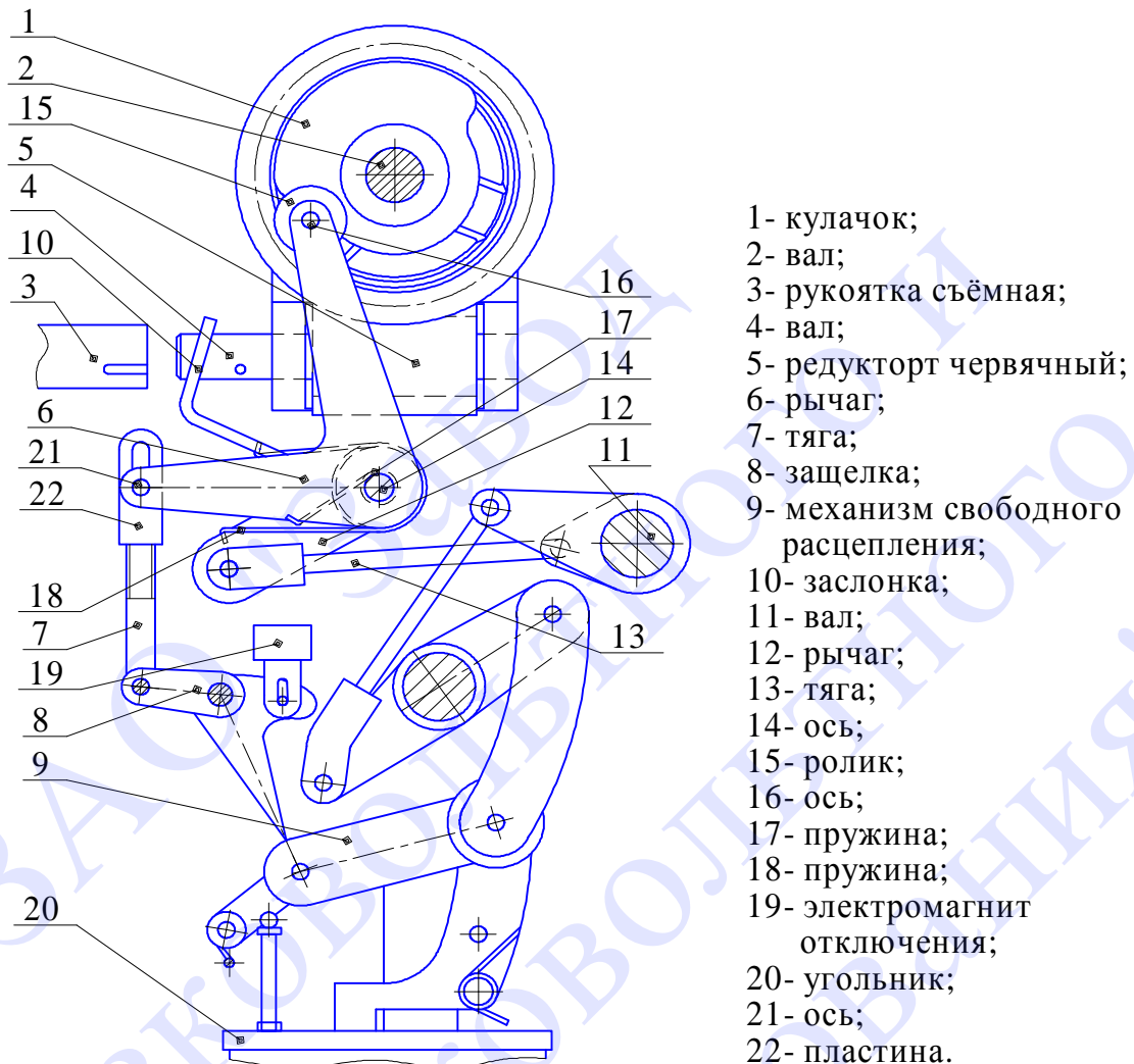
Рис.5 Блокировка выкатного элемента с выключателем типа ВМПЭ-10
