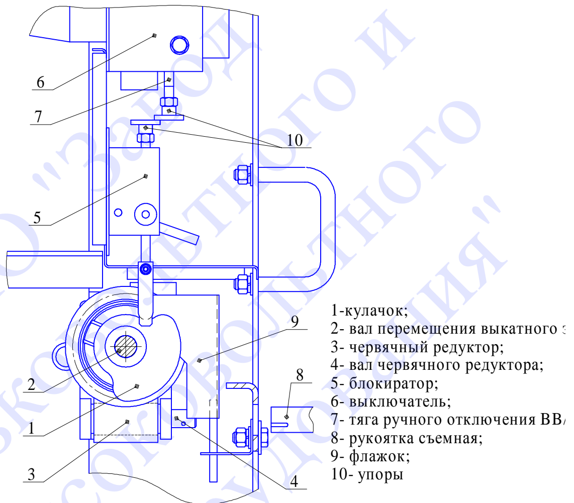
Рис.7 Блокировка выкатного элемента с выключателем ВВ/TEL-10 с нижним
