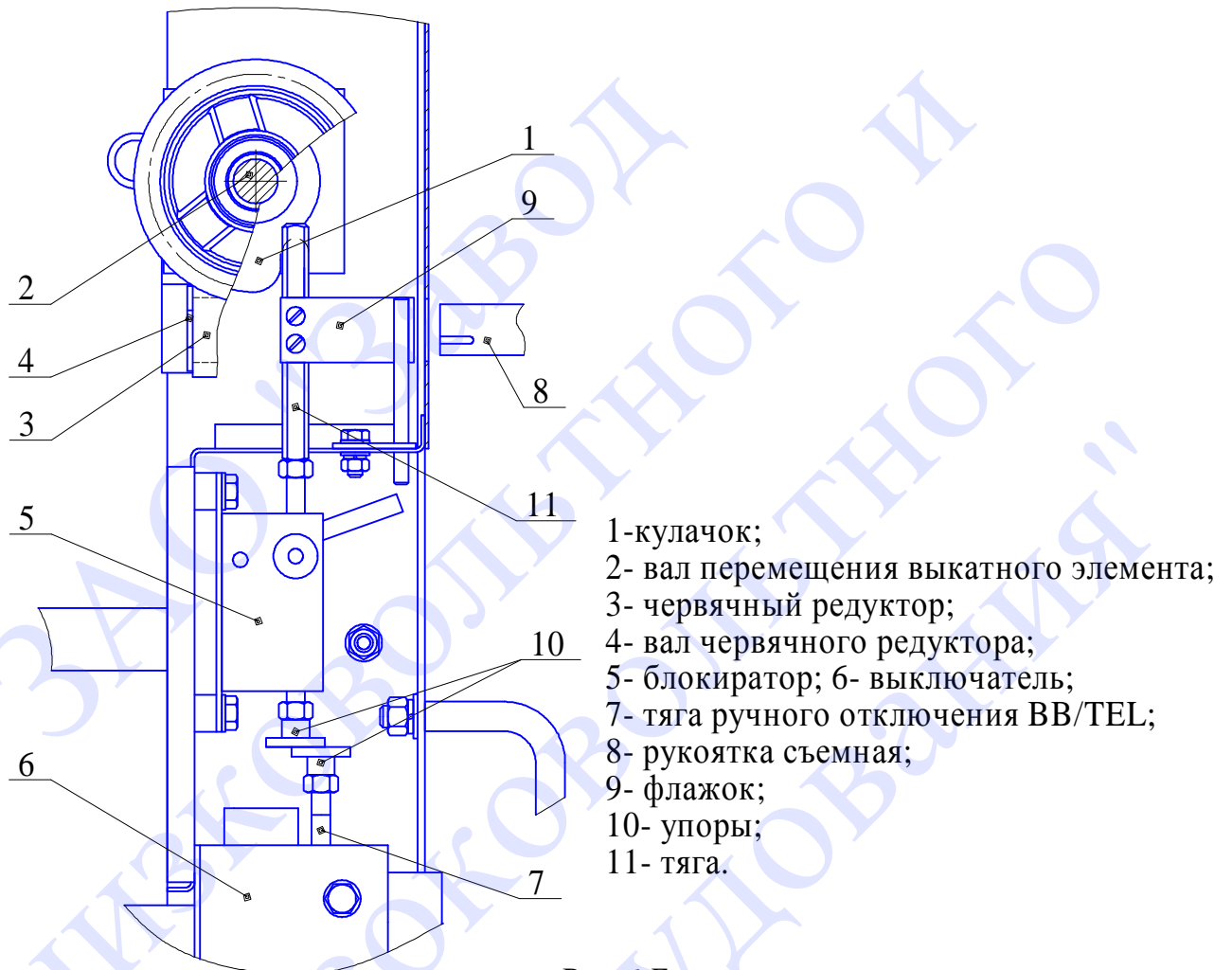
Рис.6 Блокировка выкатного элемента с выключателем ВВ/TEL-10 с верхним вкатом
