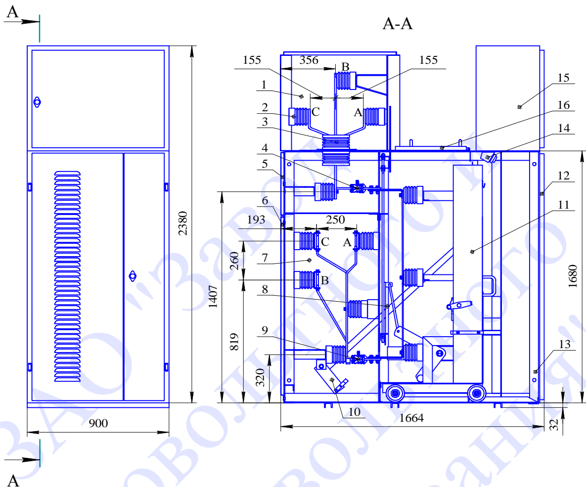
Рис.3 Шкаф с розеткой разъединителя.
