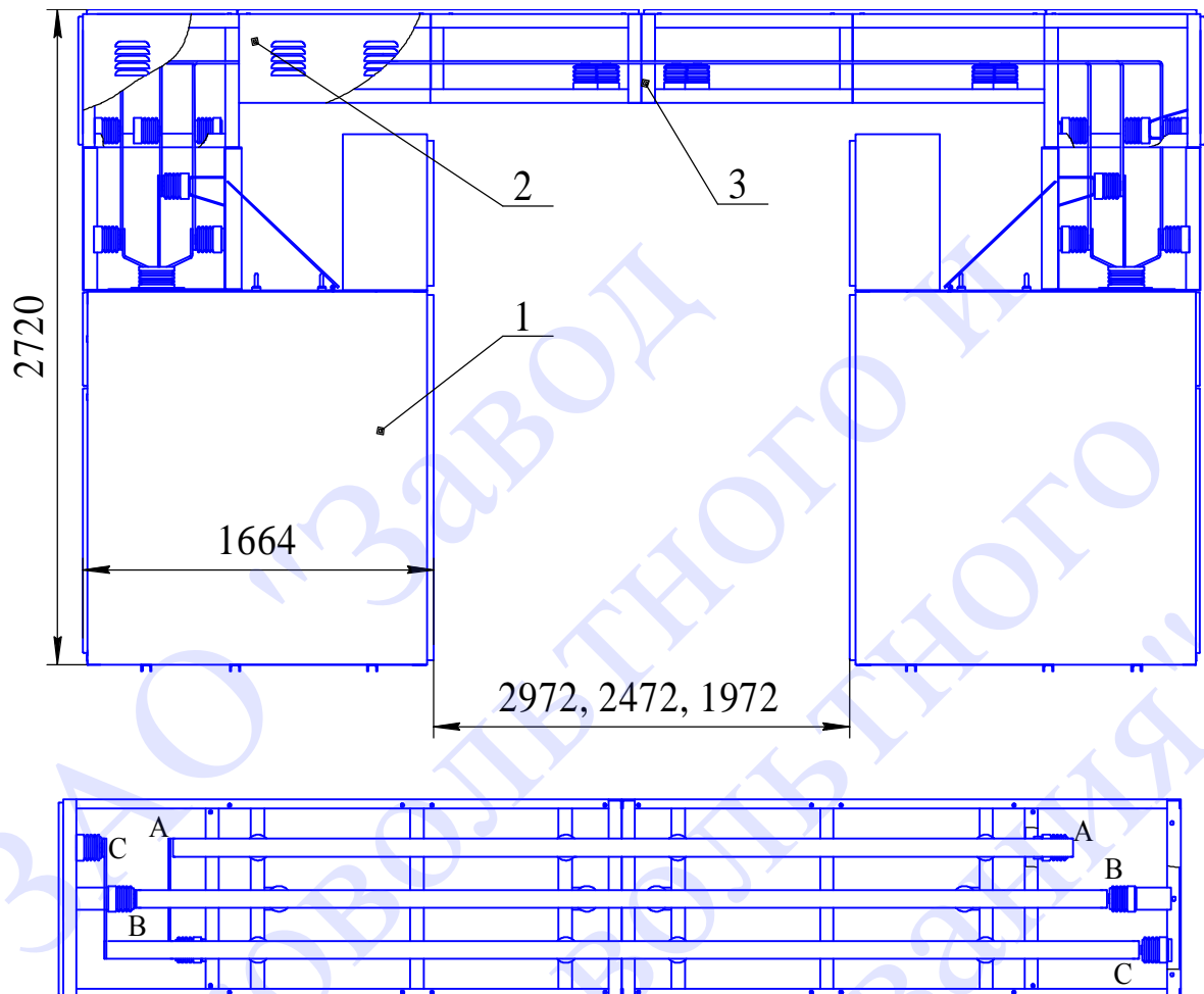
Рис. 11 Токопровод.
