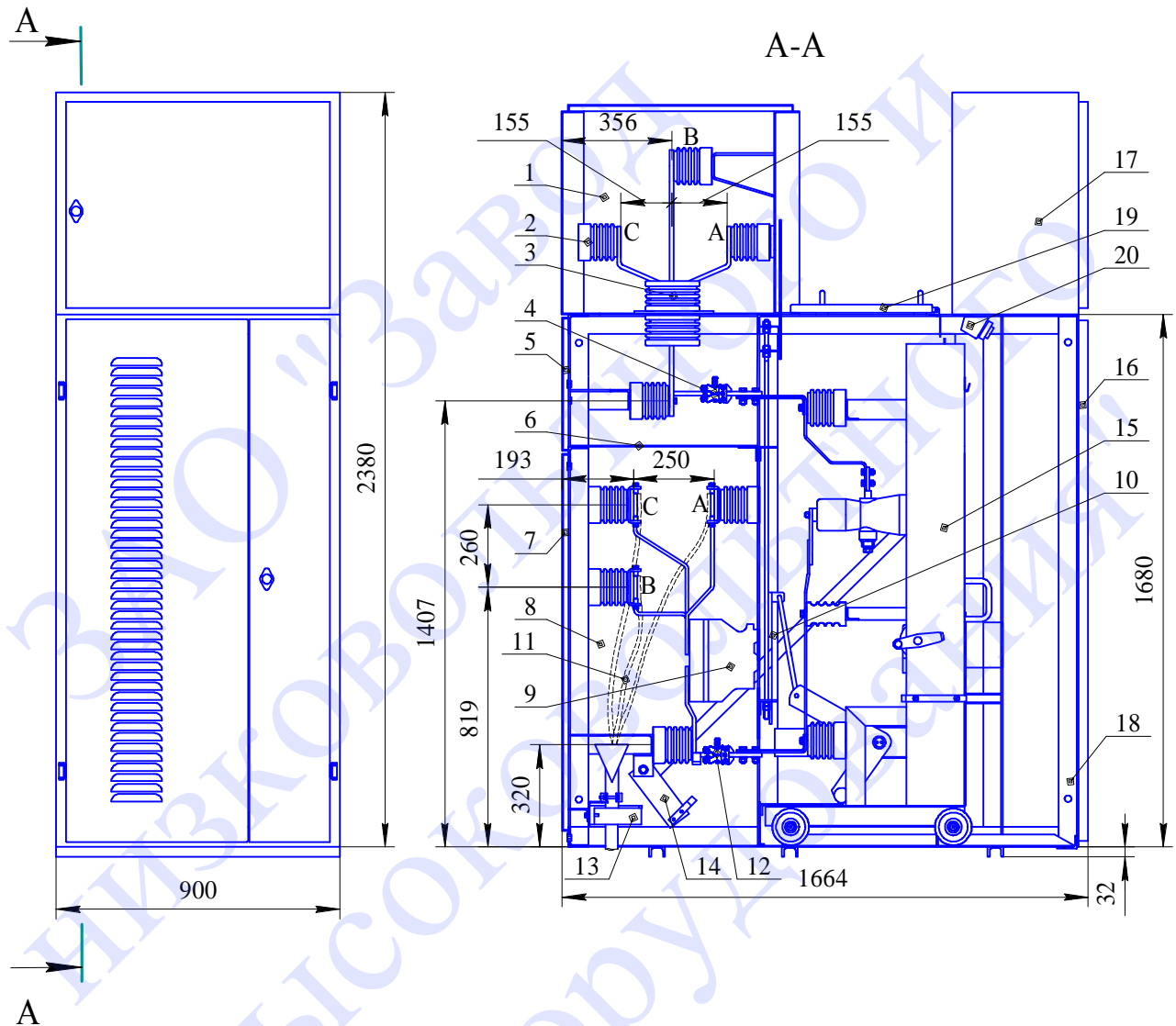
Рис.1 Шкаф с выключателем и трансформатором тока ТЛК-10 и шинным выводом влево.
