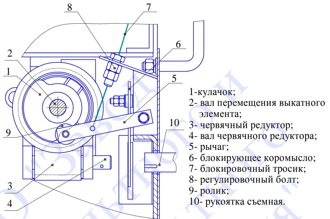
Рис. 8 Блокировка выкатного элемента с выключателем ВБМ-10.
