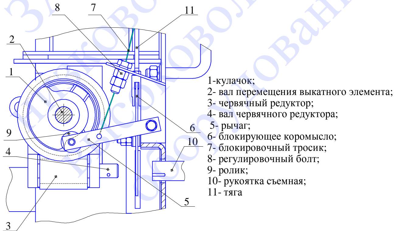
Рис. 9 Блокировка выкатного элемента с выключателем ВБЭС-10.
