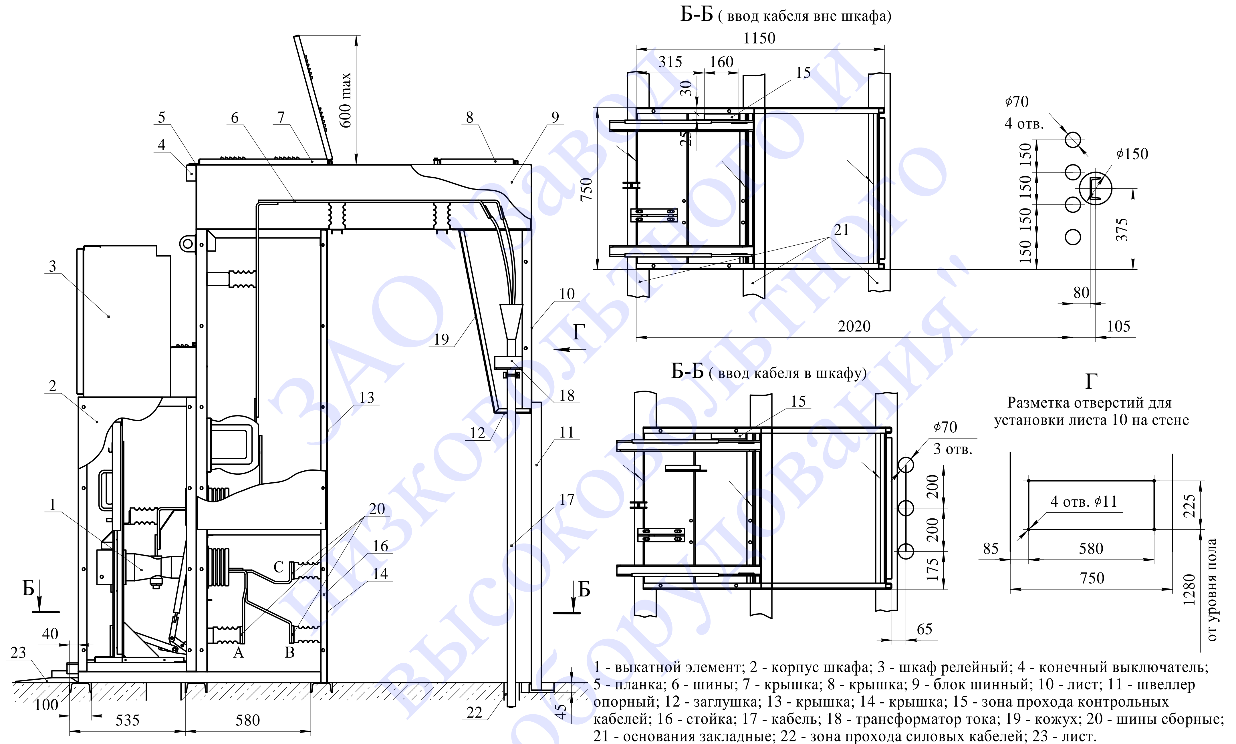
Рис. 6 Монтаж шкафов KV-02-104
