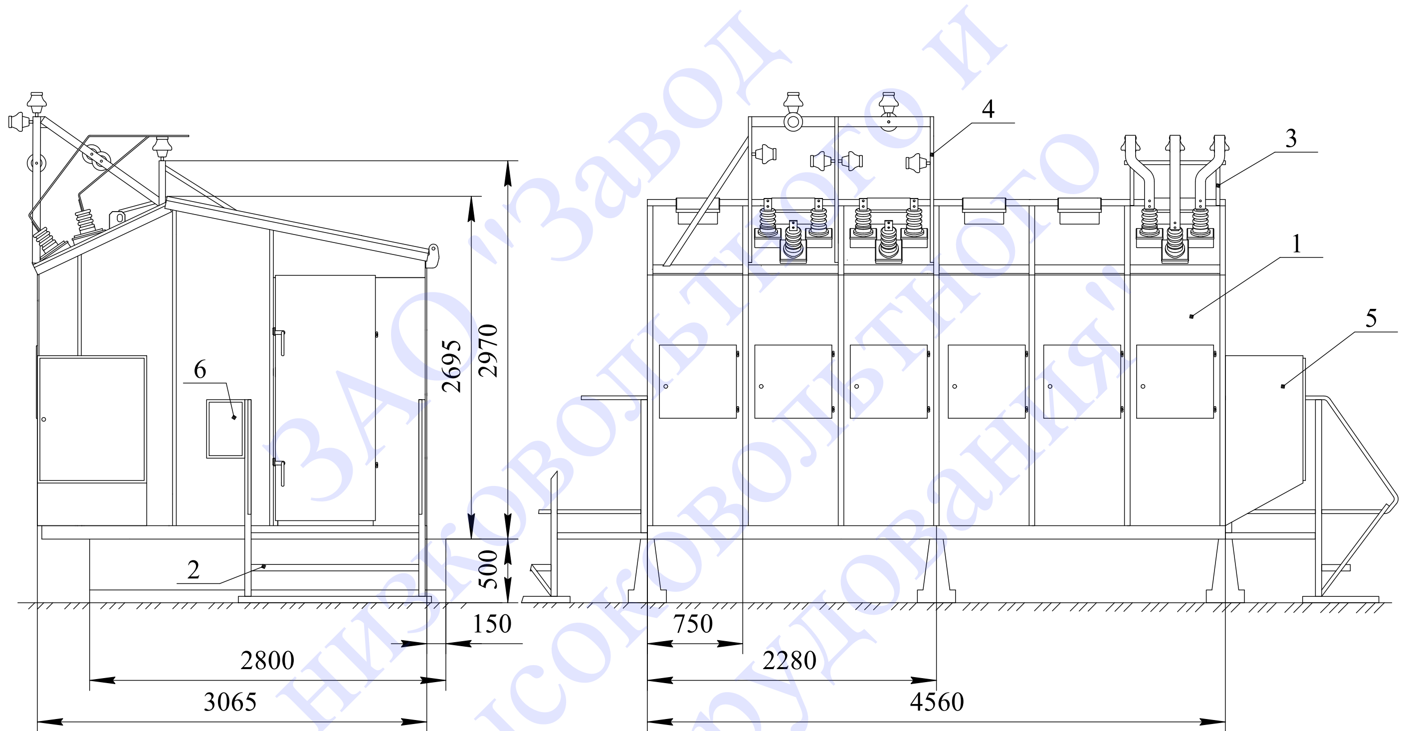
Рис. 1. Общий вид блока КРУН исполнения У1 (вариант установки на незаглубленном фундаменте): 1 - блок КРУН; 2 - лестница; 3 - кронштейн ввода; 4 - кронштейн линии; 5 - шкаф с трансформаторами напряжения; 6 - подставка инвентарная
